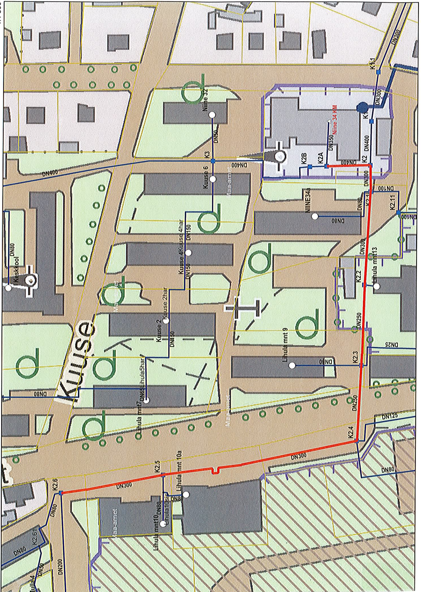
Lisa 1 projekteerimistingimustele nr 32-12 ASENDISKEEM
